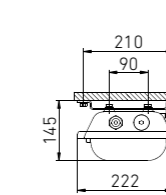
Монтажные кронштейны
