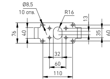
Монтажная скоба
