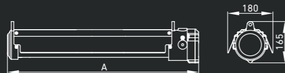
Габаритные размеры
